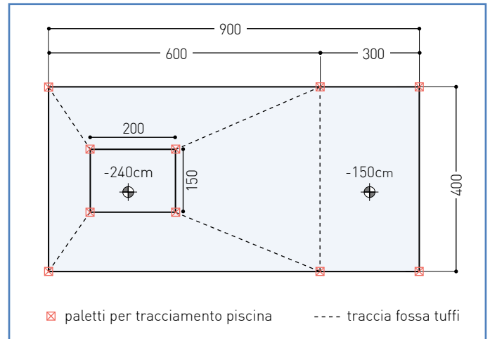
Sequenza di tracciatura della fossa tuffi - fase 2
