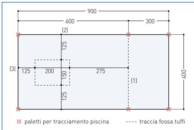
Sequenza di tracciatura della fossa tuffi - fase 1
