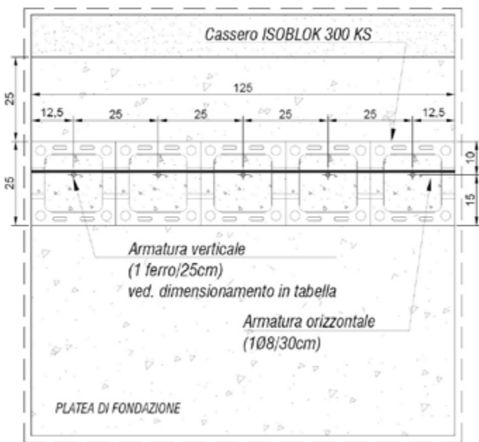
Disposizione dei ferri di armatura verticali
