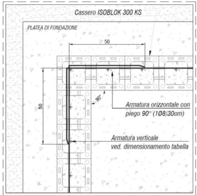
Dettaglio sovrapposizione armatura orizzontale
