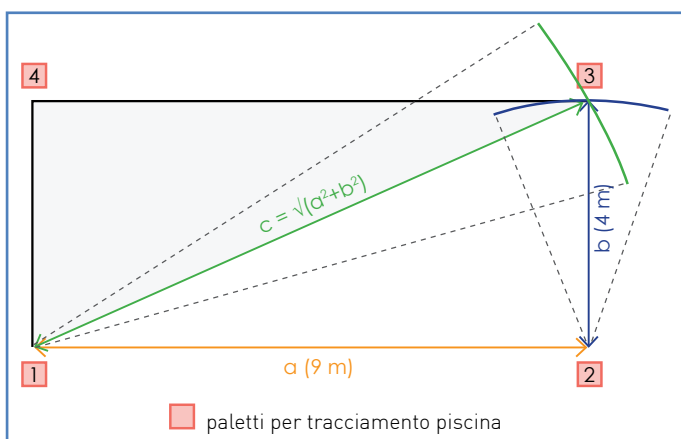
Sequenza di tracciamento della forma (vista dall'alto)
