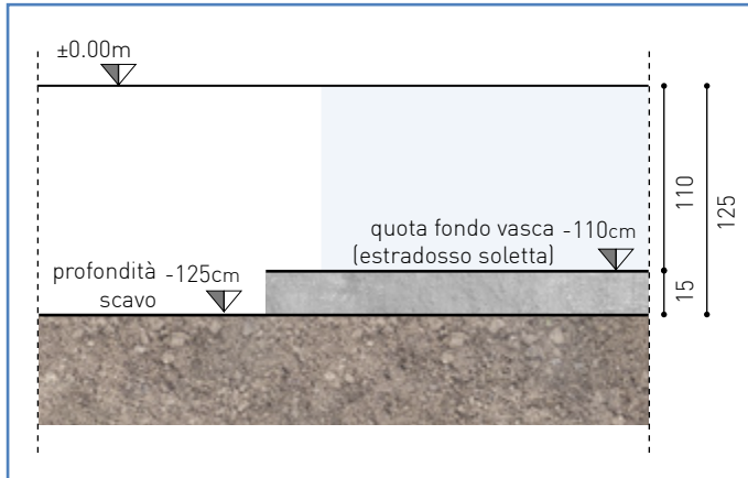
Esempio: profondità dello scavo (vista in sezione)
