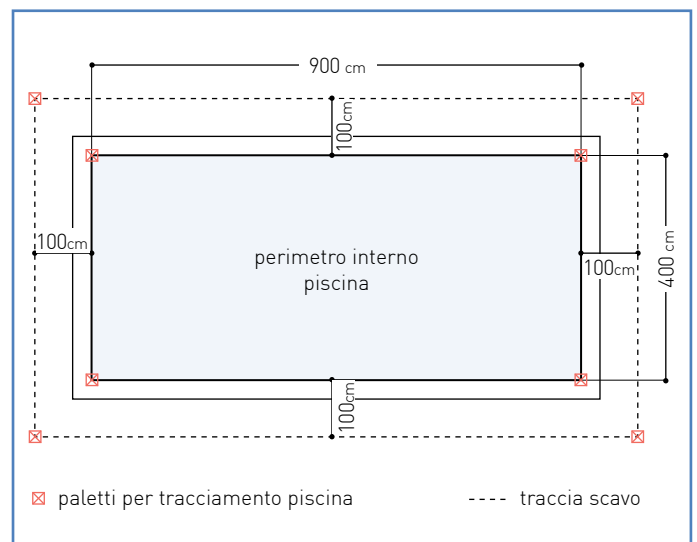
Schema della vasca e dello scavo (vista dall'alto)
