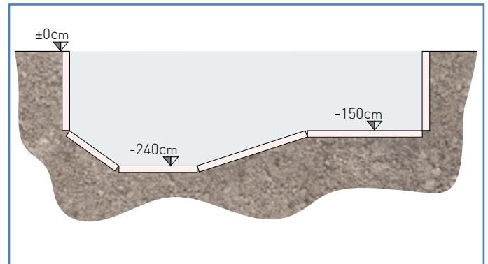
Fossa tuffi (sezione trasversale)
