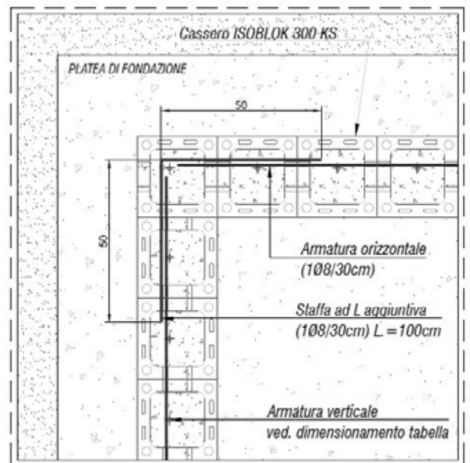
Dettaglio sovrapposizione armatura orizzontale con staffa L
